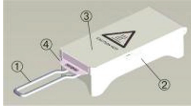
VarioSmoker für den Garraum mit Versorgungskabel
