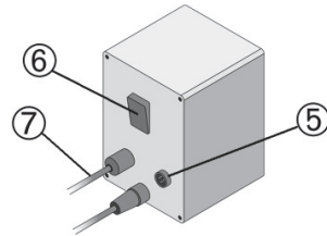
パリオ・スモーカー (庫内設置用) と電源ケーブル
